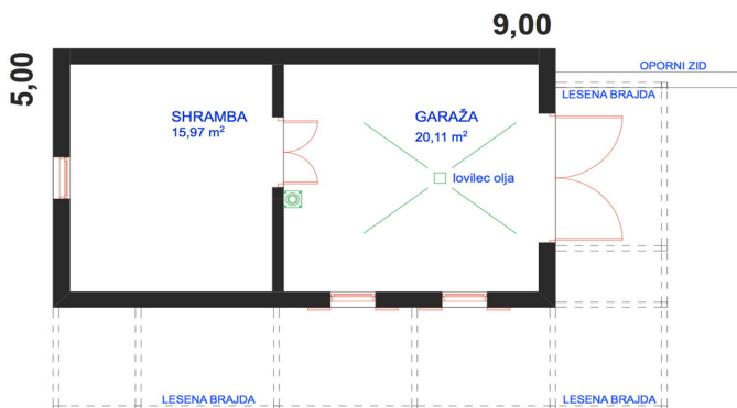
KLET
