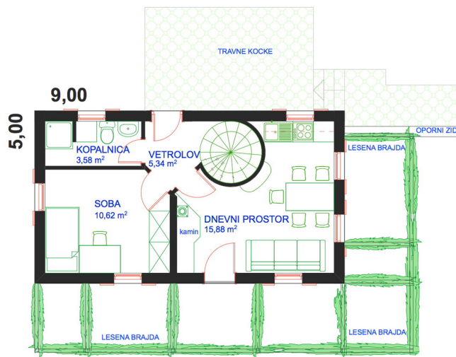
PRITLIČJE
